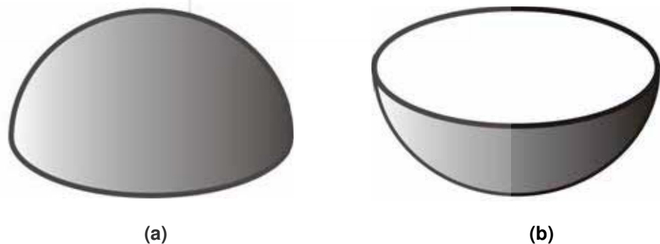
Fig. 10.14: a) Dome; and b) Basin.
