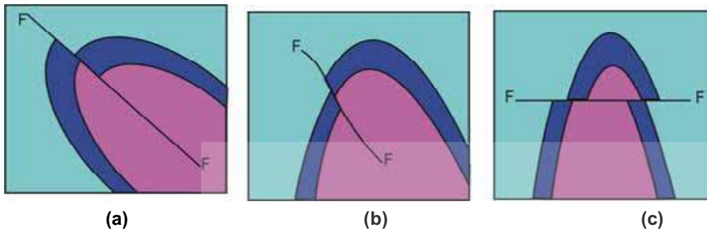
Fig. 11.6: a) Longitudinal fault; b) Transverse fault; and c) Tear fault.
