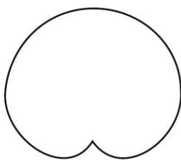
(d) r = a + b \sin \theta
