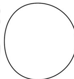
(h) \frac{a}{b} > 2 (Convex)
